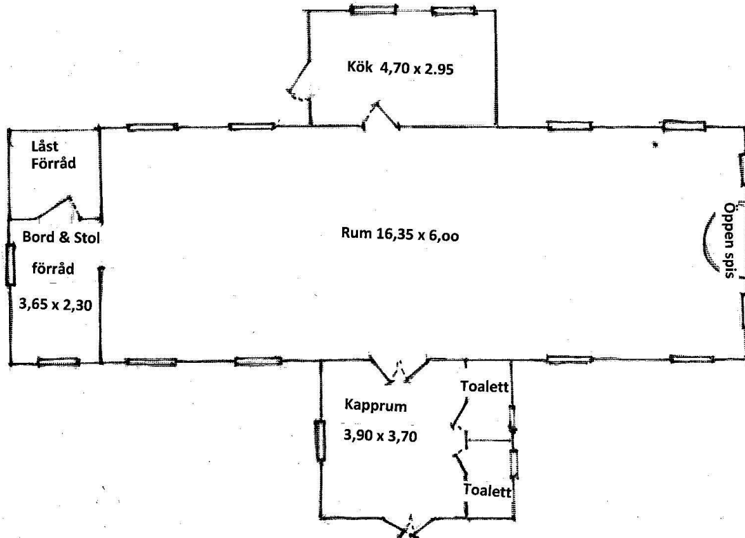
Ringparksstugan Skala 1:100
